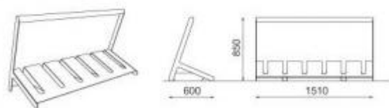
struttura d'acciaio, portabiciclette a 6 posti
