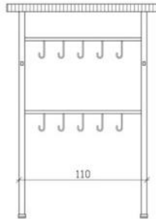
VISTA FRONTALE
